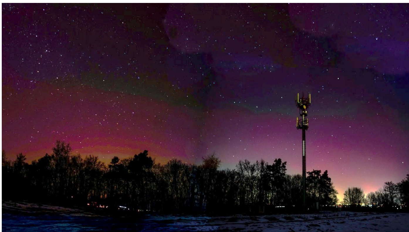
Polární záře v pondělí 19. ledna 2026 nad Novými Ouholicemi (fot. Martin Čech)
